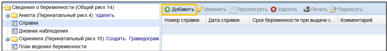
Рисунок 7 – Кнопка "Добавить"
